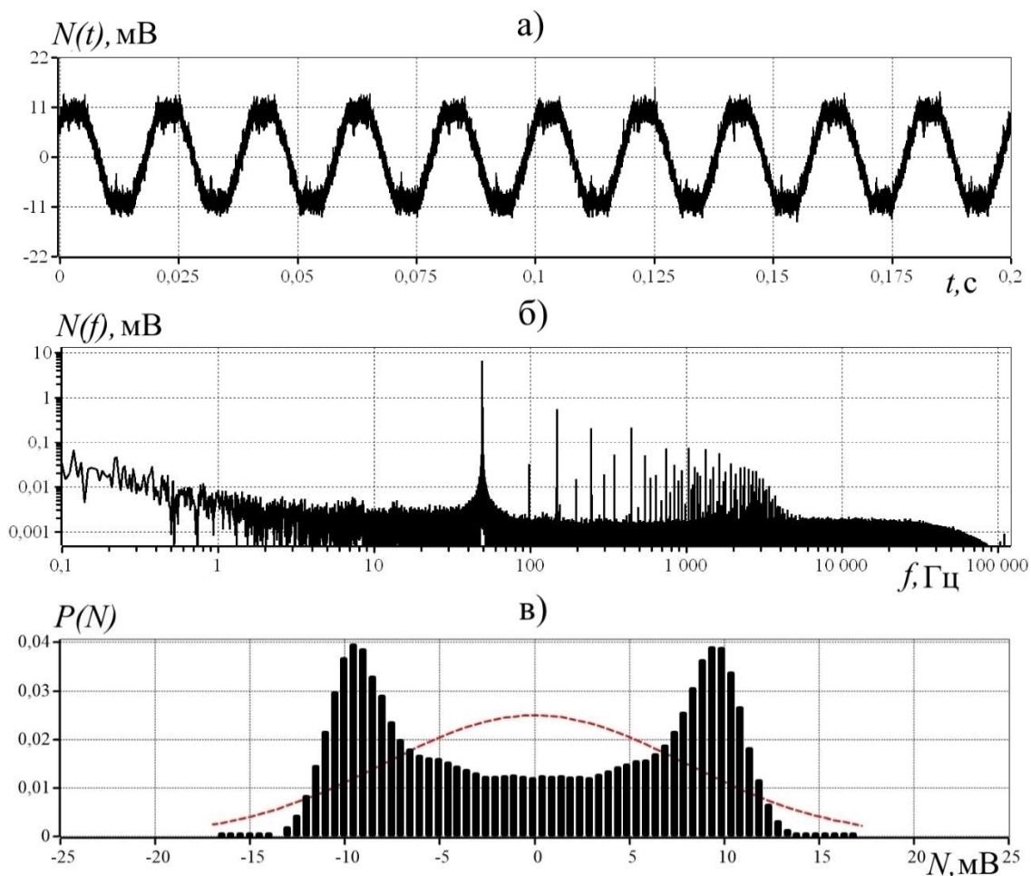
Рис. 1. Первичные данные регистрации шума (фрагмент) - а), его частотный спектр - б) и плотность вероятности распределения амплитуд помех и шумов - в) в измерительном сеансе.
