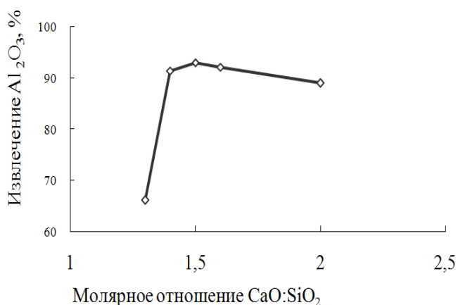
Рис. 2. Влияние дозировки оксида кальция на извлечение глинозема
