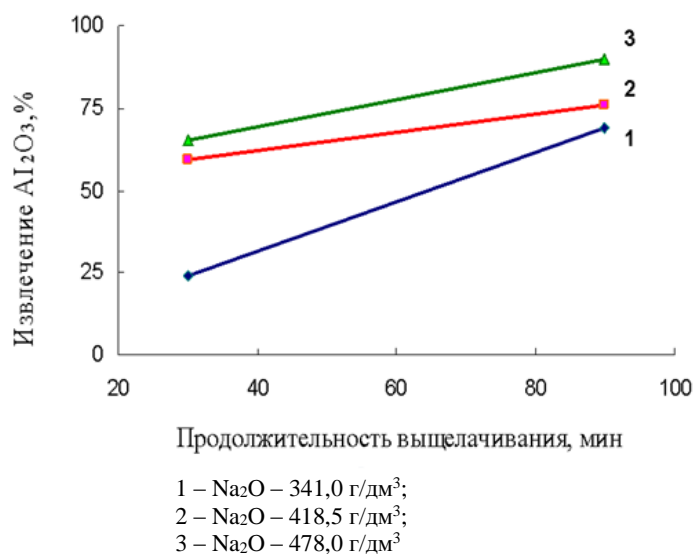
Рис. 1. Влияние концентрации раствора на извлечение глинозема
