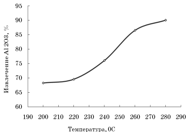
Рис. 3. Влияние температуры выщелачивания на извлечение глинозема
