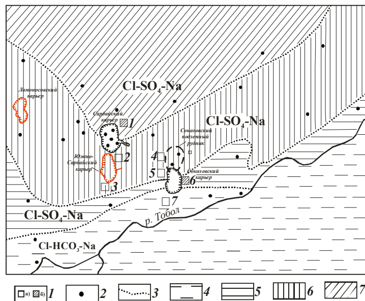
Рис. 4. Гидрохимическая схема эоценового водоносного горизонта района Соколовского и Сарбайского железорудных месторождений: 1- водоотливные стволы дренажных шахт: а) – действующие, б) - ликвидированные (1- Северная Сарбайская (ликвидирована в марте 2000 года), 2- Южная Сарбайская, 3- Южная Сарбайская Вентиляционная, 4- Вспомогательная СПР, 5-Южная Вентиляционная Соколовского карьера и подземного рудника, 6-Южная I Соколовского карьера (ликвидирована в апреле 1991 года), 7-Южная II Соколовского карьера); 2-гидрохимические точки опробования; 3- границы зон с различной минерализацией и химическим составом; 4-7-зоны с различной минерализацией, г/дм 3 (4-до 1; 5-2-3; 6-3-4; 7-свыше 4).
