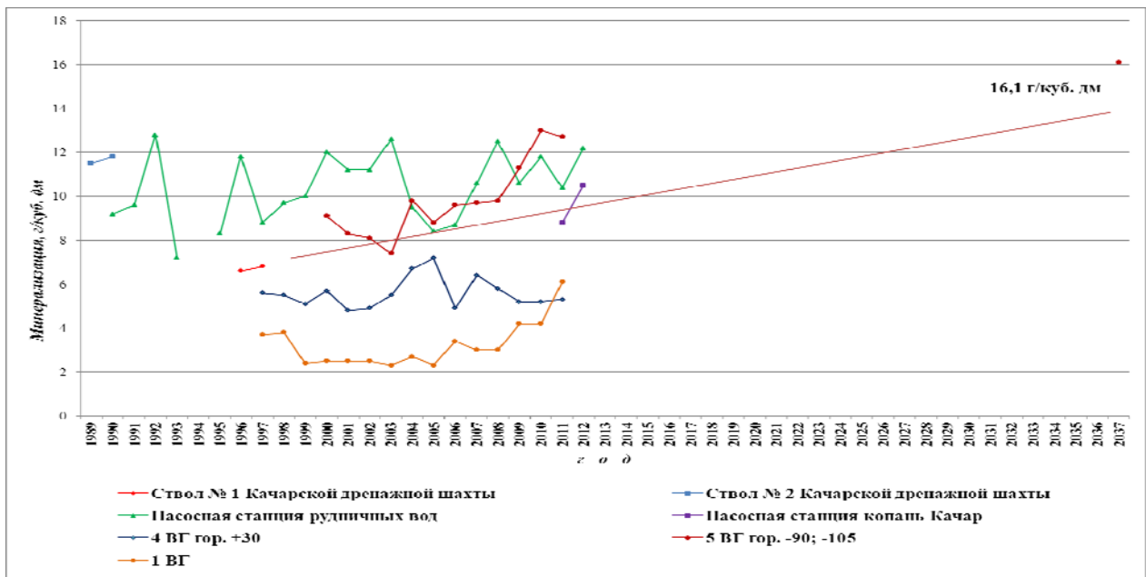
Рис. 2. Динамика изменения минерализации по водоотливным комплексам и водоносным горизонтам Качарского месторождения за 1989-2012 гг.
