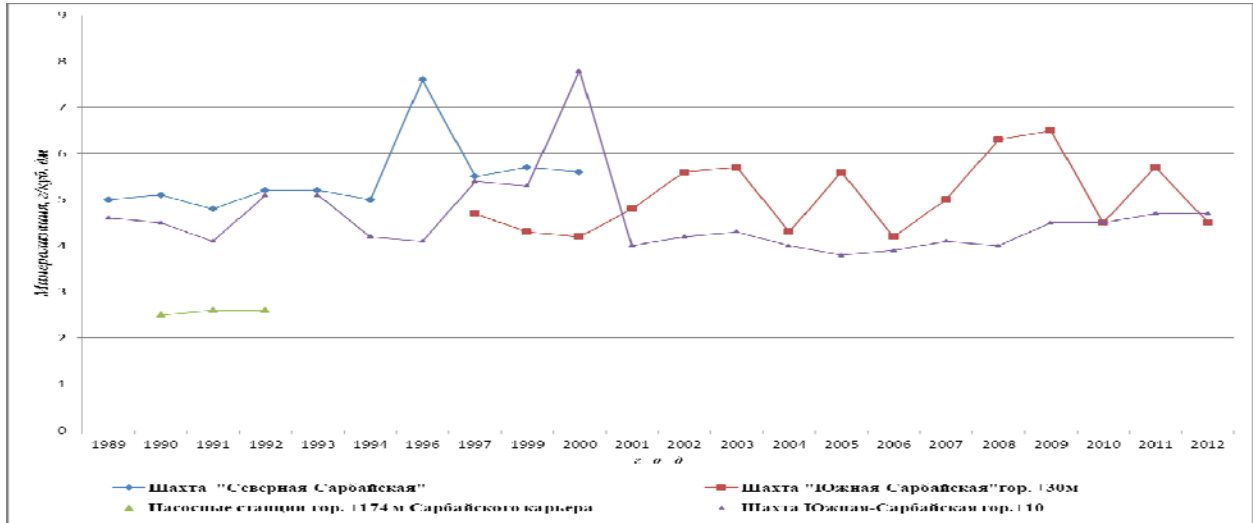
Рис.1. Динамика изменения минерализации по водоотливным комплексам Сарбайского месторождения за 1989-2012 гг.
