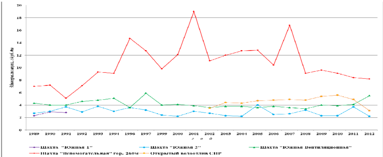
Рис. 3. Динамика изменения минерализации по водоотливным комплексам Соколовского месторождения за 1989-2012 гг.
