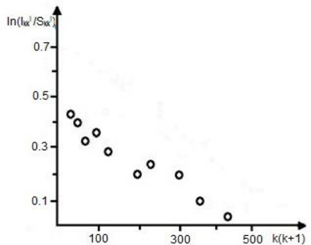
Рис. 2. Зависимость величины \ln(I_{kkI} / S_{kkI}) от k(k+1) для вращательной структуры молекулярного иона азота.
