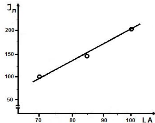
Рис.3. Зависимость интенсивности вращательной линии
