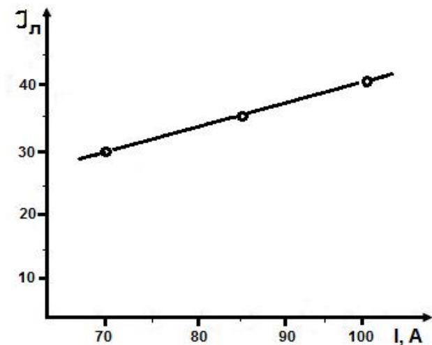
Рис. 2. Зависимость интенсивности вращательной линии R7 ( B^2 \Sigma_u^+ \rightarrow X^2 \Sigma_g^+, 0-0 ) от силы тока на расстоянии H=10 мм от среза сопел. Интенсивность дана в относительных единицах.
