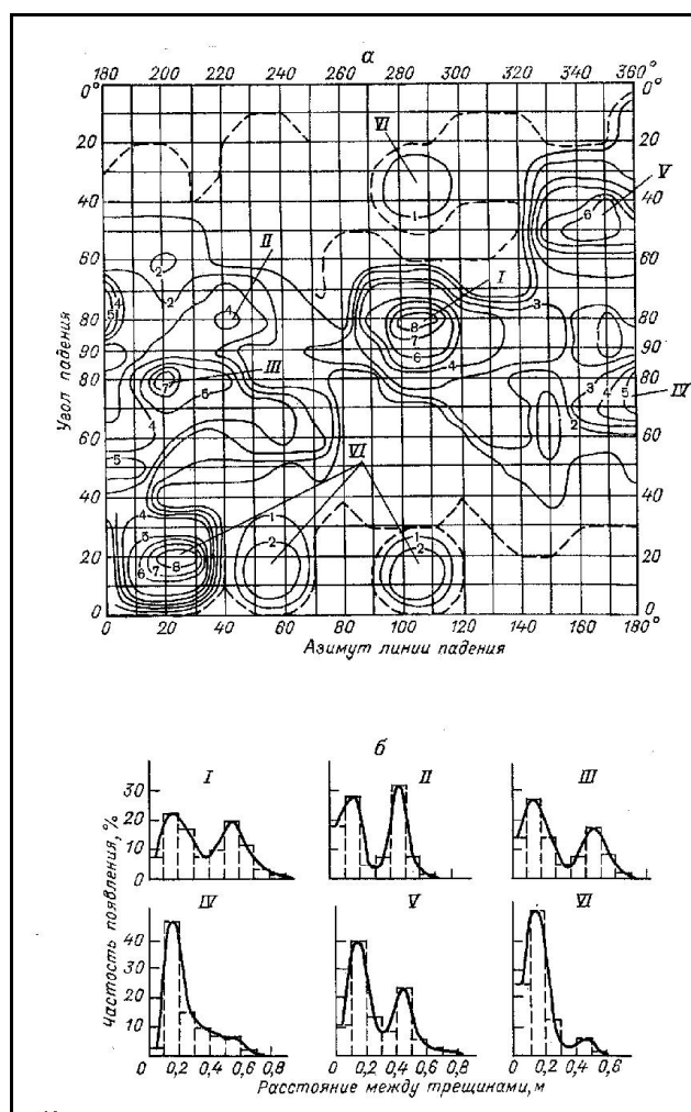
Рис.2. Системы трещин:
