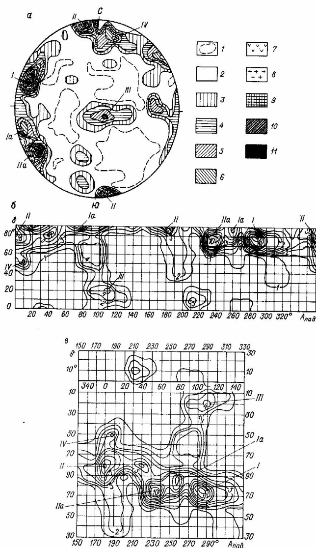
Рис 1. Типы диаграмм трещиноватости массива в изолиниях.
