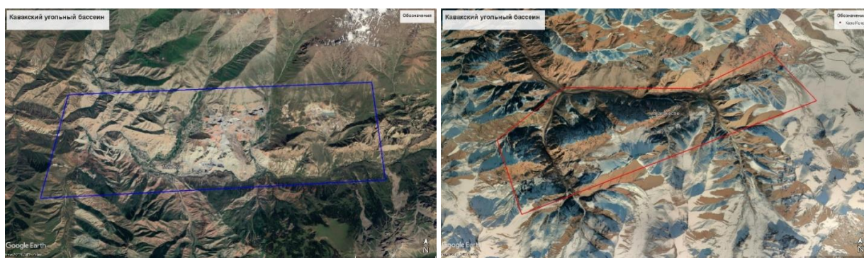
Рис. 1. Кавакский угледобывающий бассейн: а) Мин-Куш, б) Кара-Кече.
