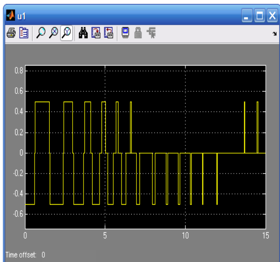
Рис. 7. Закон управления u_1(t)
