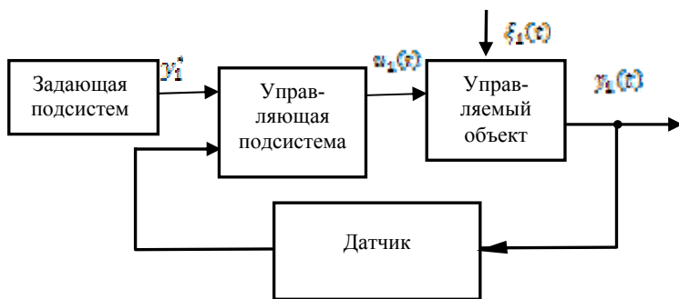
Рис. 1. Общая структура системы регулирования.
