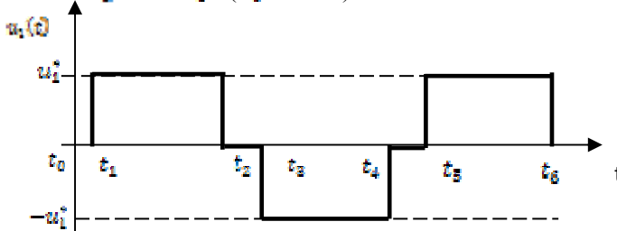
Рис. 2. Управляющие импульсы
