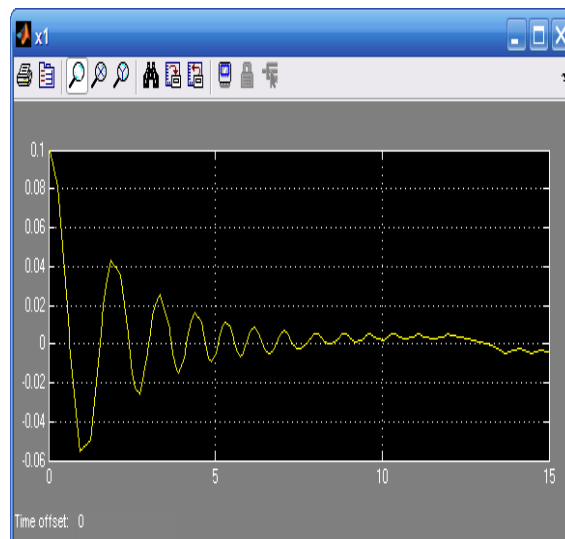
Рис. 8. Переходный процесс по ошибке управления e_1(t)
