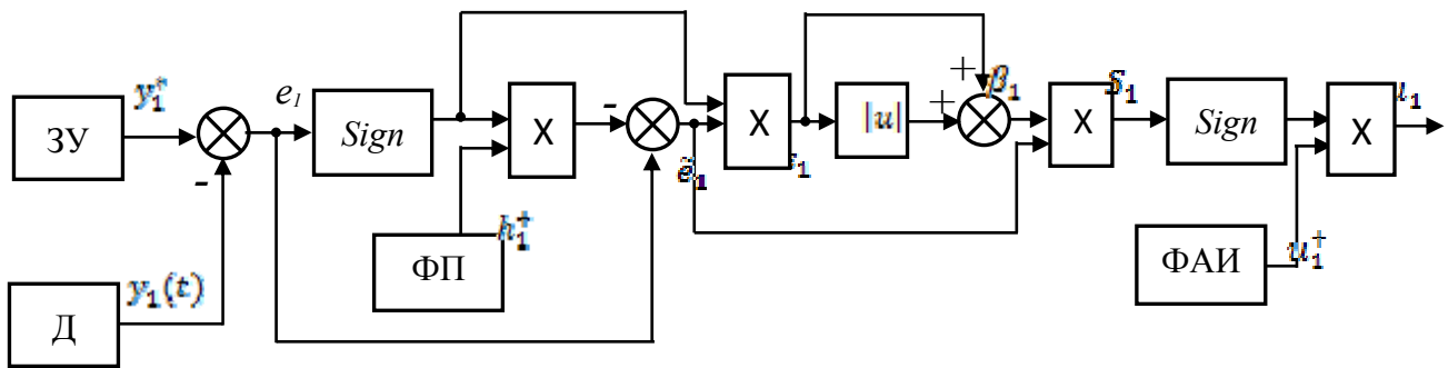
Рис. 3. Структура регулятора САУ
