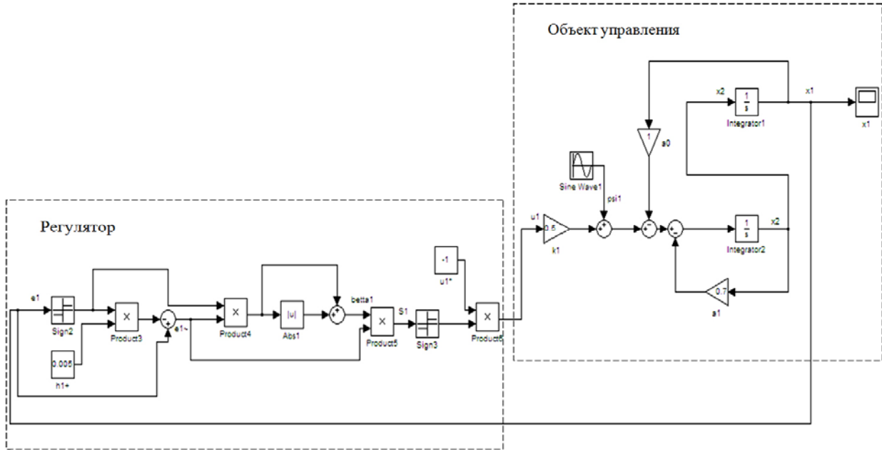
Рис. 4. Схема компьютерного моделирования САУ
