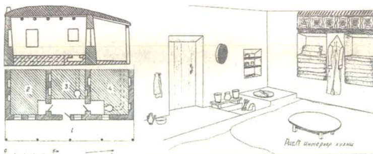
Рис. 2 Традиционный тип уйгурского жилища «коржун» построенный в нач. XX в. План. Разрез. С. Панжим Панфиловский р-н. Талды- курганской обл. Интерьер кухни /по А.Б.Зульярову
